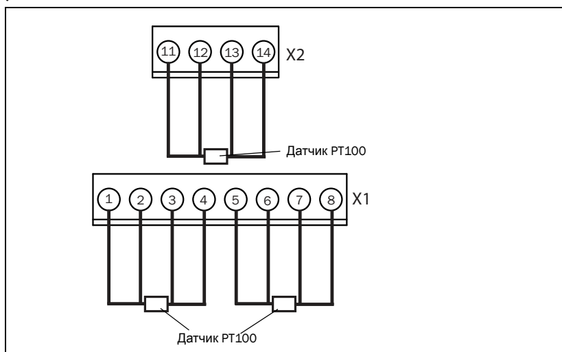
Рис. 8 Подключение датчиков PT100.
