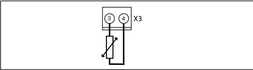
Рис.4 Подключение датчика PTC
