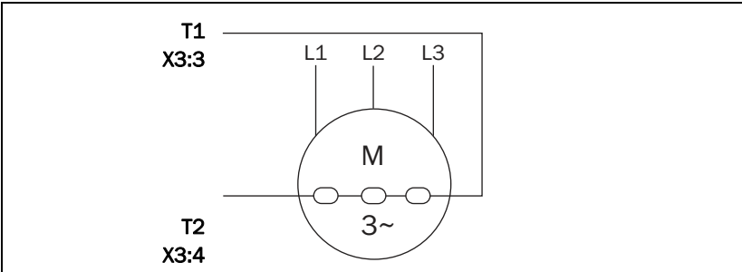
Рис.5 Пример применения с тремя датчиками PTC, подключенными последовательно.
