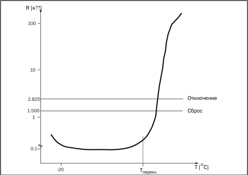
Рис.3 Типичная кривая датчика PTC
