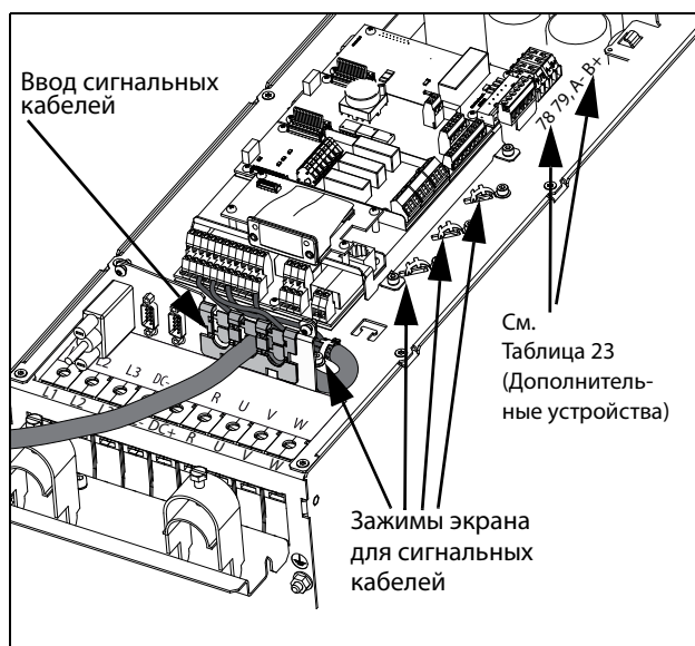
Рис. 62 Подключение кабелей управления, модели VFX 48-060 до 48-105, с размером корпуса D2 и модели 69-033 — 69-058 с размером корпуса D2(69).
