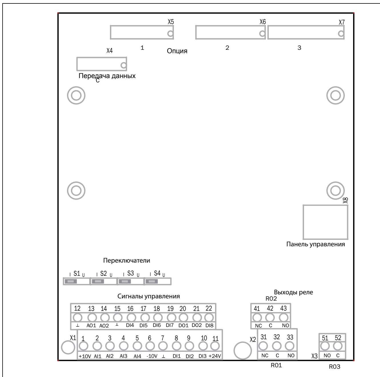
Рис. 56 Внешний вид платы управления
