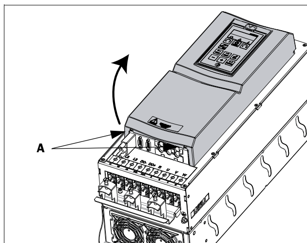
Рис. 29 Снятие передней крышки на корпусе с размером C2–F2 и FA2 (принципиальная схема)
