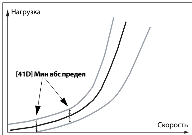
Рис. 123 Кривая нагрузки R с минимальным абсолютным пределом
