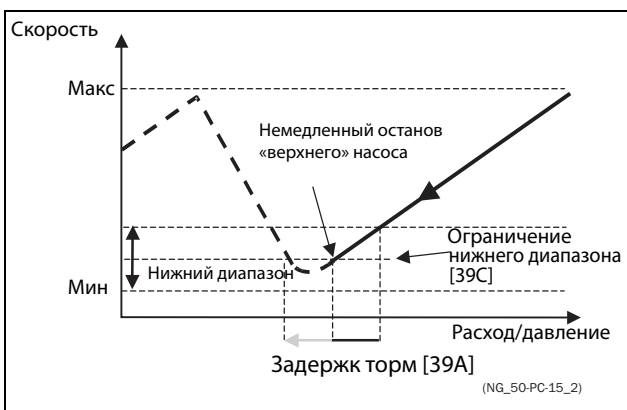
Рис. 118 Ограничение нижнего диапазона
