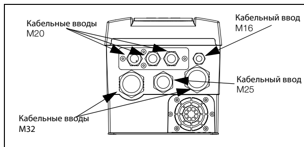
Рис. 6 Кабельный интерфейс для подключения электрической сети, электродвигателя и управления, Emotron VFX моделей 48/52-003 — 018 (размер корпуса B).
