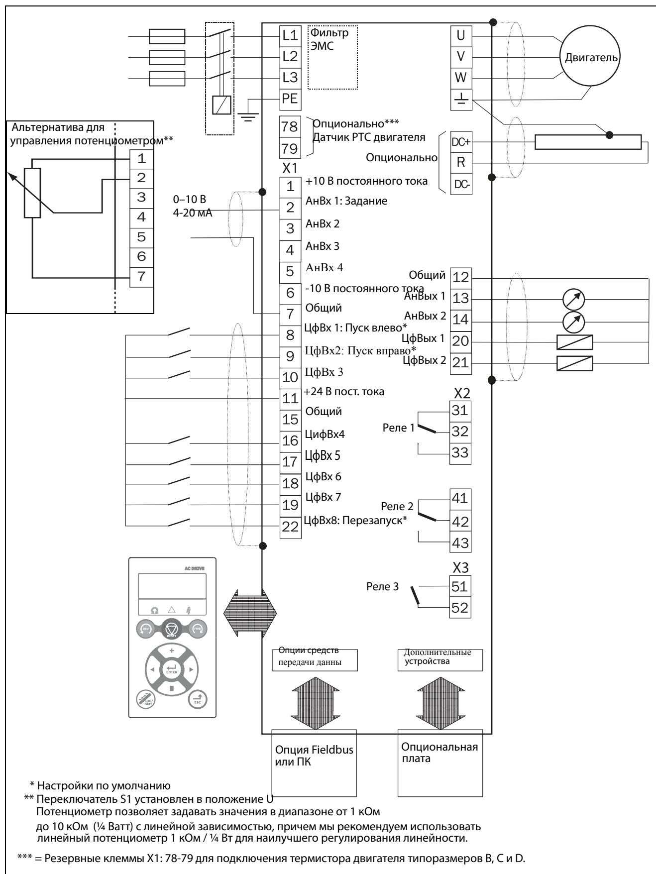
Рис. 57 Пример подключения
