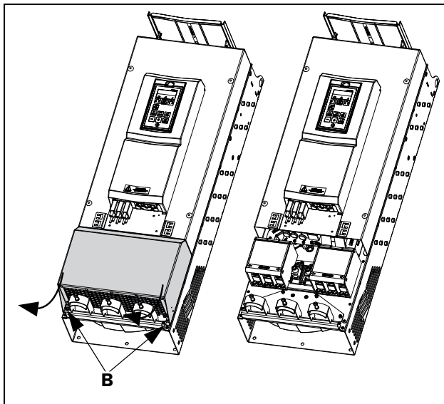
Рис. 30 Ослабьте два винта и снимите нижнюю крышку (принципиальная схема)
