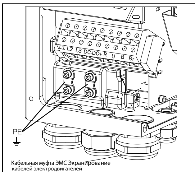
Рис. 32 Подключение сетевого питания и двигателя модели 026-046, размер корпуса C.
