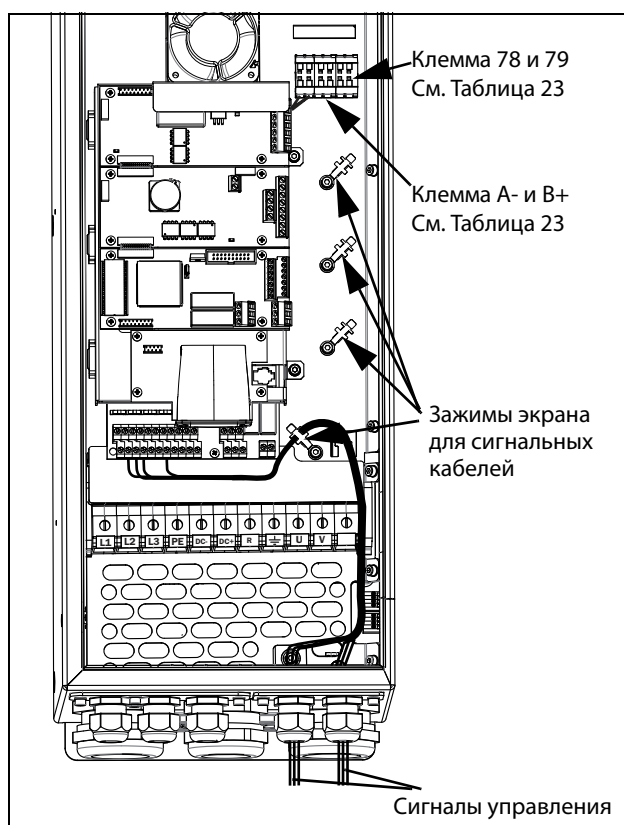
Рис. 61 Подключение кабелей управления, VFX модели 061 — 074 с размером корпуса D и модели 69-033 — 69-058 с размером корпуса D(69).
