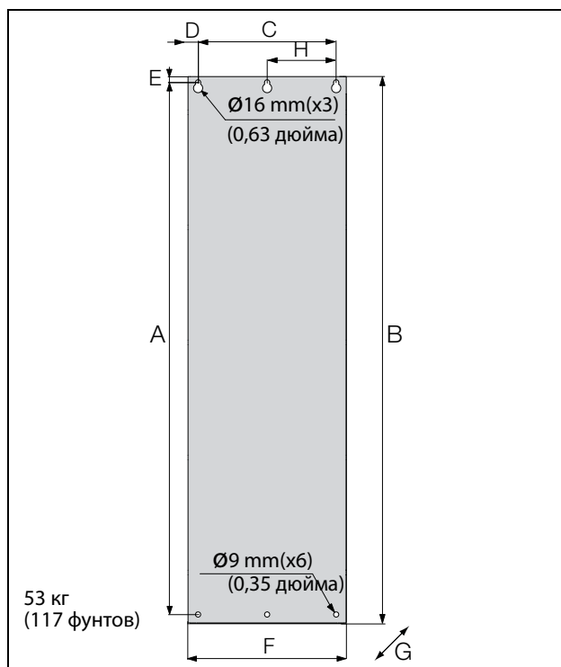
Рис. 22 Устройство VFX/ моделей от 48-142 до 48-171 (размер корпуса E2).
