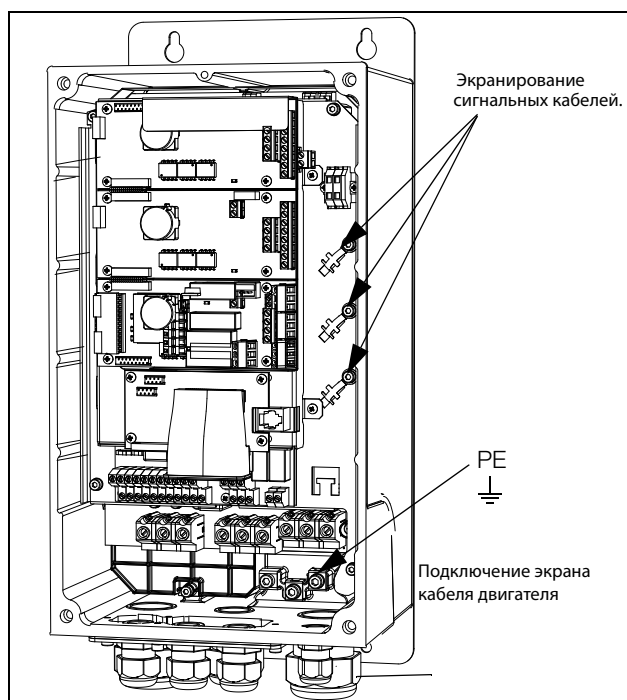
Рис. 41 Экранирование кабелей.
