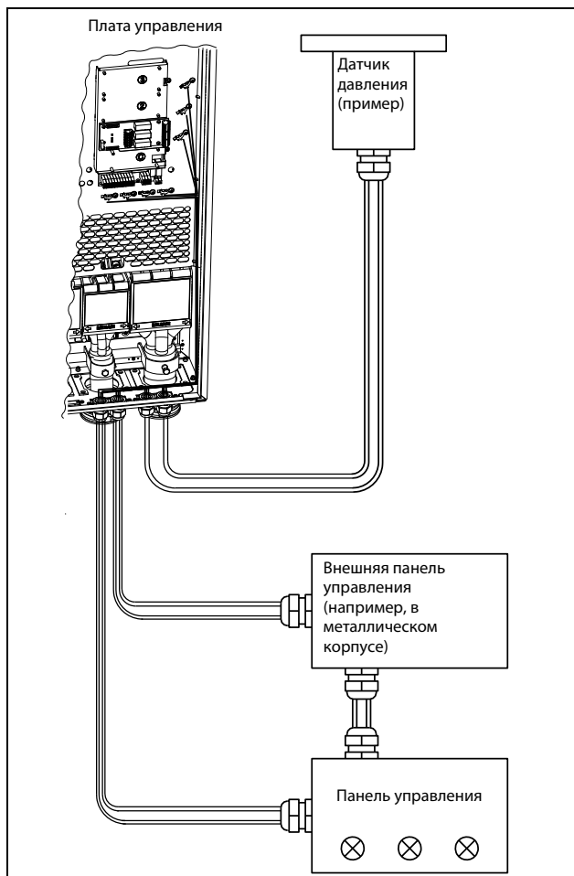
Рис. 65 Электромагнитное экранирование кабелей управляющих сигналов.
