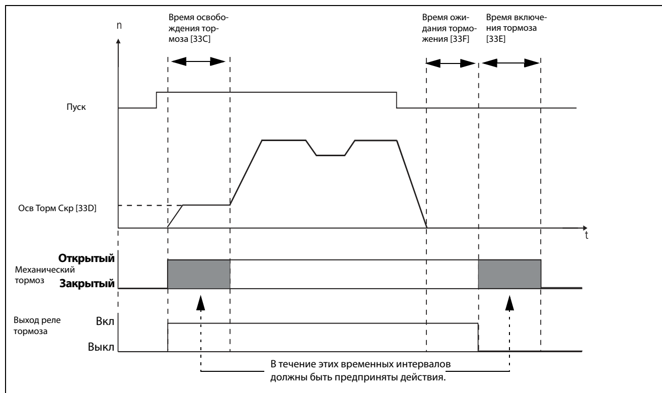
Рис. 103 Функции торможения
