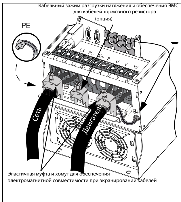
Рис. 36 Подключение сетевого питания и двигателя, модели от 48-060до 48-105, размер корпуса D2 и модели 69-033 — 69-058, размер корпуса D2(69).
