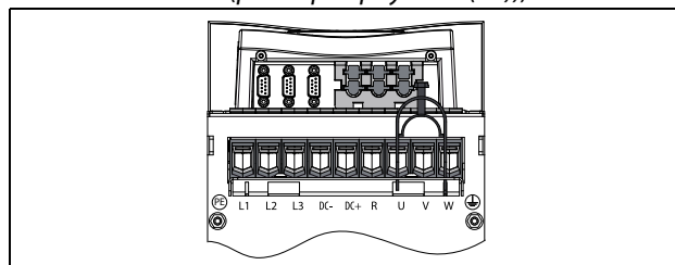
Рис. 17 Вид снизу, устройство Emotron VFX моделей с 48-060 по 48-105 (размер D2), моделей с 69-033 по 69-058 (размер корпуса D2(69)), с кабельным интерфейсом для подключения электрической сети, электродвигателя, опции DC+/DC-, тормозного резистора и управления.
