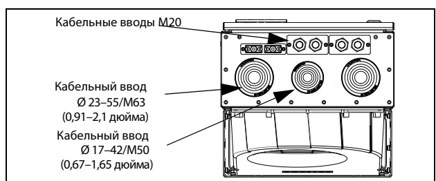
Рис. 21 Кабельный интерфейс для подключения электрической сети, электродвигателя, DC+/DC-, тормозного резистора и связи, устройство Emotron VFX моделей с 48-210 по 295 (размер корпуса F), устройство Emotron VFX моделей с 69-082 по 200 (размер корпуса F69).
