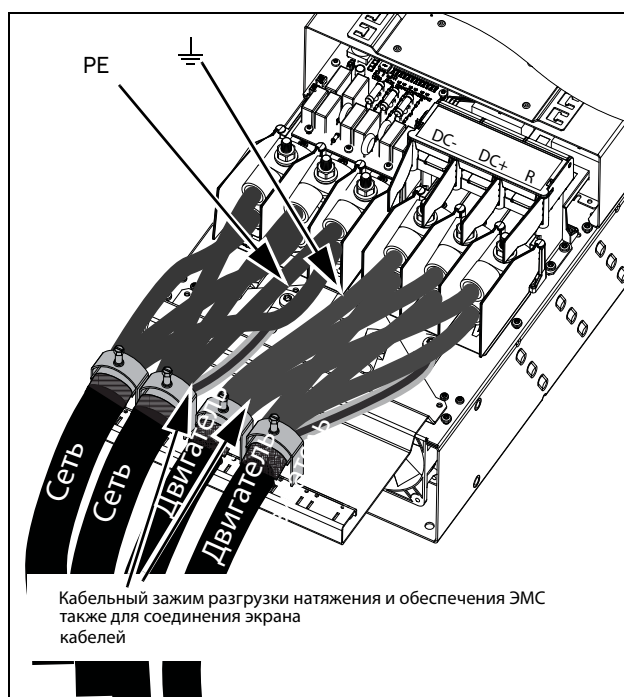
Рис. 39 Подключение сетевого питания и двигателя модели 48-365-20 (размер корпуса FA2) с дополнительными клеммами для опции DC-, DC+ и тормоза (принципиальная схема)
