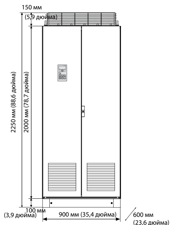
Устройство Emotron VFX48: модели 600–750 (размер корпуса I) Устройство Emotron VFX69: модели 430–595 (размер корпуса I69)
