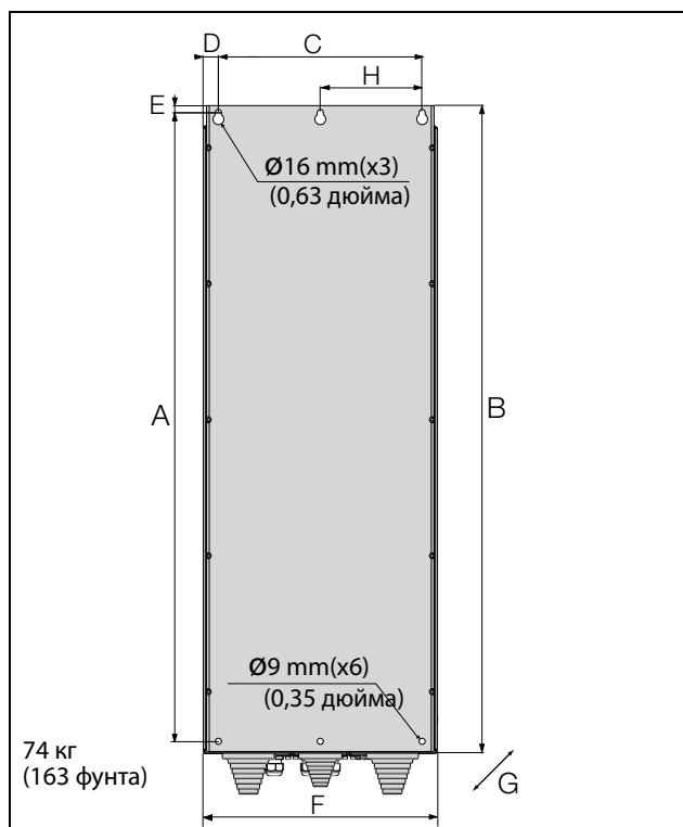
Рис. 20 Устройство Emotron VFX моделей с 48-210 по 295 (размер корпуса F), Устройство Emotron VFX моделей с 69-82 по 200 (размер корпуса F69).
