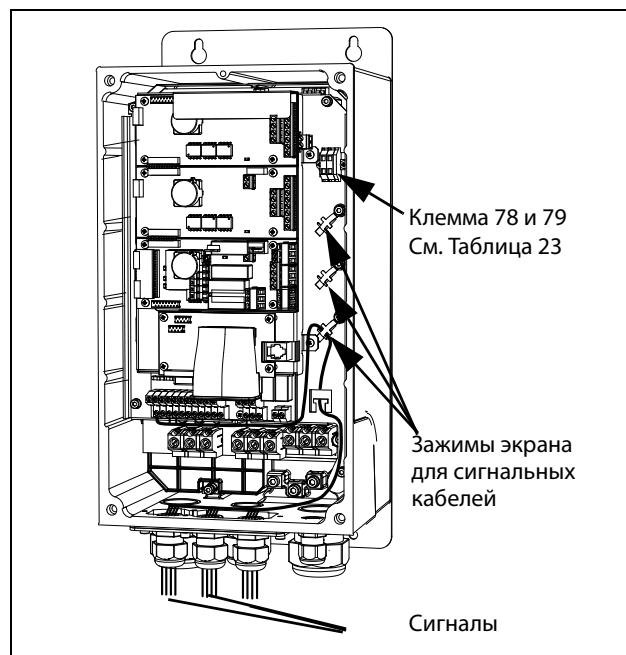
Рис. 58 Подключение кабелей управления, VFX модели от 003 до 018, типоразмер В.
