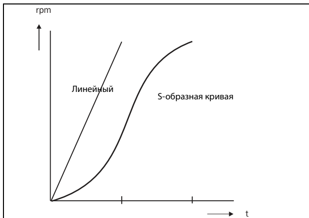
Рис. 101 Форма кривой разгона
