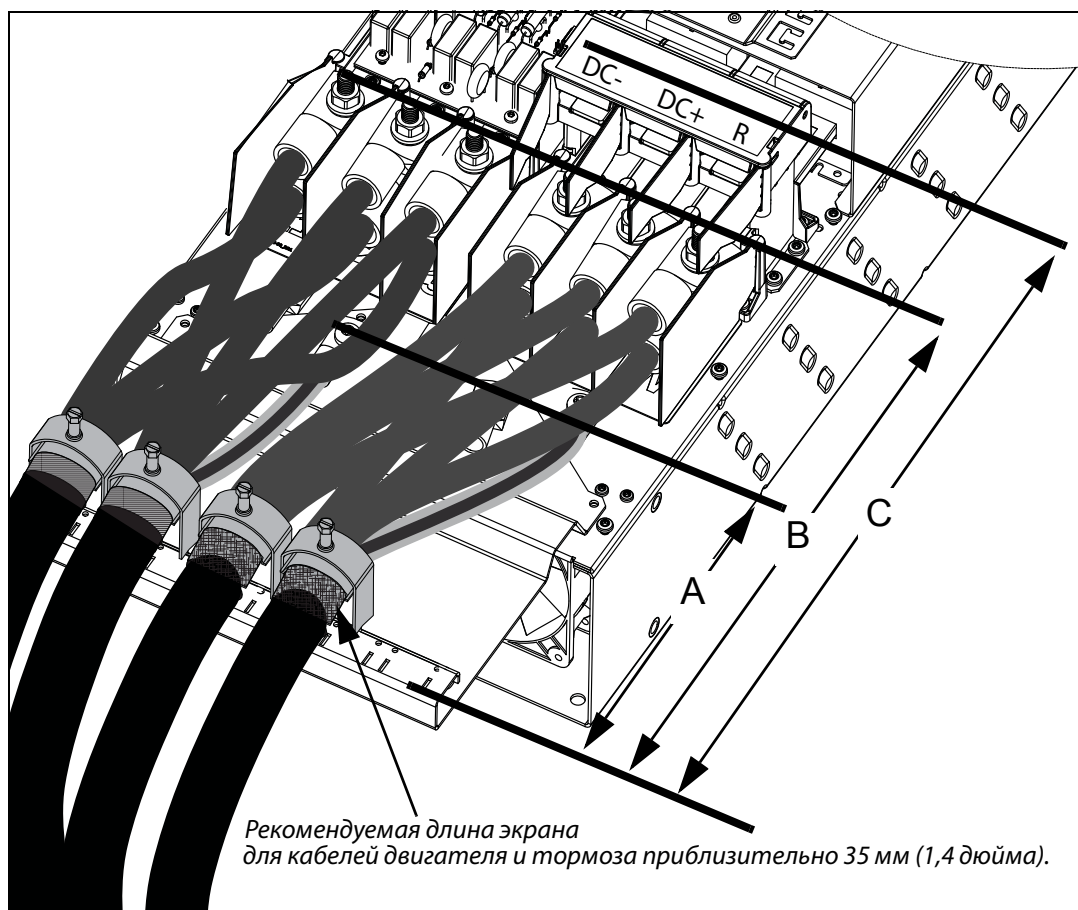
Рис. 54 Расстояния от кабельного зажима до соединительных болтов размера FA2
