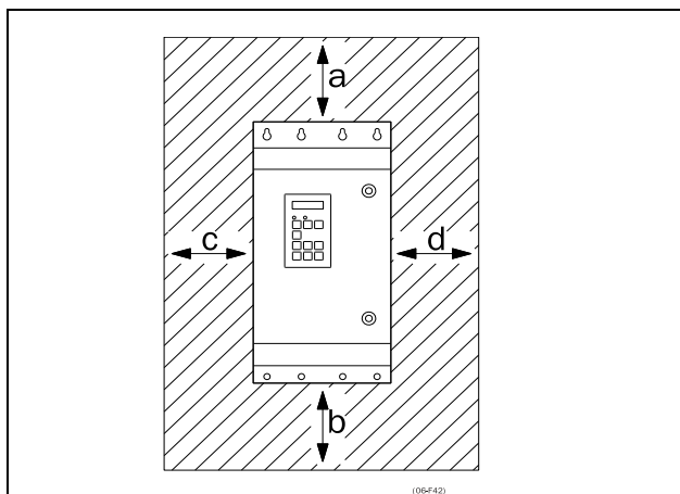
Рис. 4 Монтаж преобразователей частоты типов с 002 по 3K0
