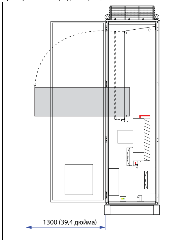
Рис. 28 Рекомендуемое свободное пространство перед шкафом преобразователя частоты.
