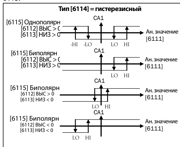
Рис. 136 Основные функции компаратора для «Тип [6114] = гистерезис» и «Полярный [6115]».
