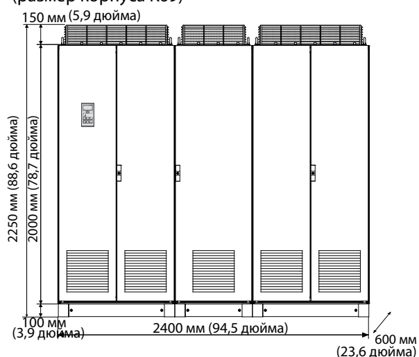
Устройство Emotron VFX48: модель 2K0 (размер корпуса M) Устройство Emotron VFX69: модель 1K6 (размер корпуса M69)
