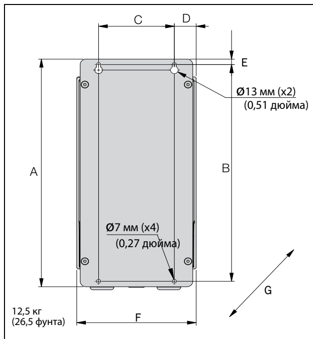
Рис. 5 Устройство Emotron VFX моделей с 48/52-003 по 018 (размер корпуса B).
