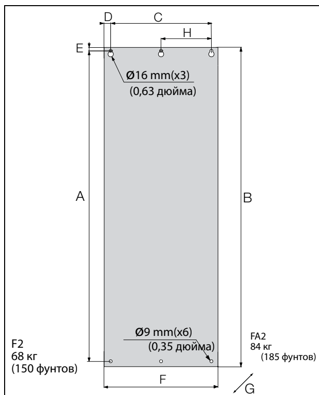
Рис. 24 Устройство VFX/ моделей от 48-205 до 48-293 (размер корпуса F2) и 48-365-20 (размер корпуса FA2).
