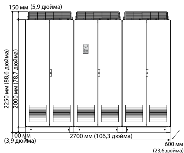
Устройство Emotron VFX48: модель 2K25 (размер корпуса N) Устройство Emotron VFX69: модель 1K8 (размер корпуса N69)
