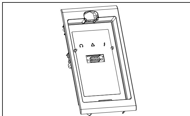
Рис. 77 Разъем RS232 под панелью управления
