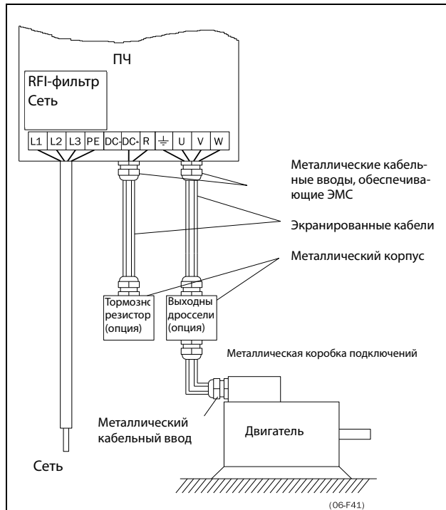
Рис. 43 Автономный преобразователь частоты
