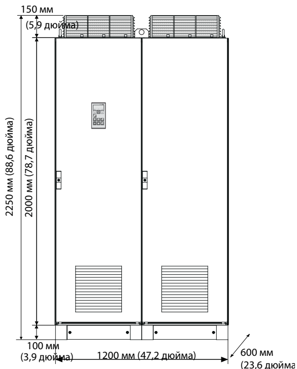
Устройство Emotron VFX48: модели от 860 до 1K0 (размер корпуса J) Устройство Emotron VFX69: модели 650–800 (размер корпуса J69)
