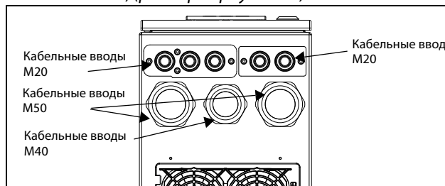
Рис. 15 Кабельный интерфейс для подключения электрической сети, электродвигателя и управления, устройство Emotron VFX моделей 48/52-061 и 074 (размер корпуса D), моделей с 69-033 по 69-058 (размер корпуса D69).
