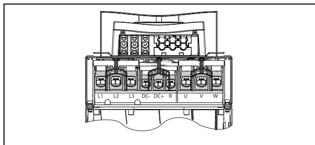
Рис. 23 Вид снизу, устройство Emotron VFX/ моделей от 48-142 до 48-293 (размер корпуса E2 и F2) с кабельным интерфейсом для подключения электрической сети, электродвигателя, опции DC+/DC-, тормозного резистора и управления (принципиальная схема).
