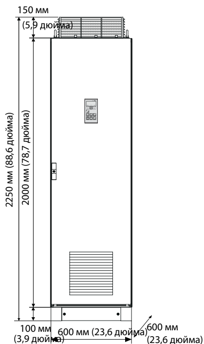
Устройство Emotron VFX48: модели от 300 до 500 (размеры корпуса G и H) Устройство Emotron VFX69: модели от 250 до 400 (размер корпуса H69)
