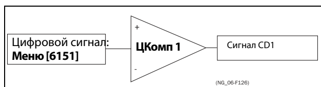
Рис. 138 Цифровой компаратор
