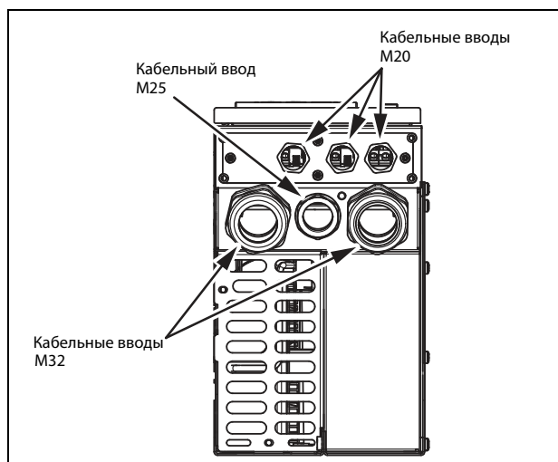
Рис. 13 Кабельный интерфейс для подключения электрической сети, электродвигателя и управления, устройство Emotron VFX моделей 69-002–025 (размер корпуса C69).
