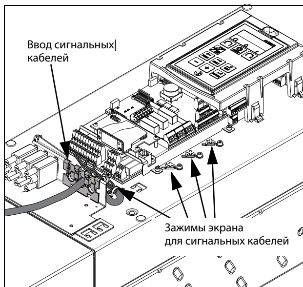
Рис. 64 Подключение кабелей управления, модели VFX 48-142 до 48-365, размеры E2, F2 и FA2 (принципиальная схема).
