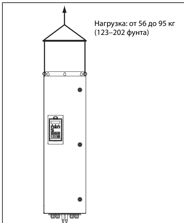
Рис. 2 Подъем для преобразователей частоты моделей с -090 по -365.
