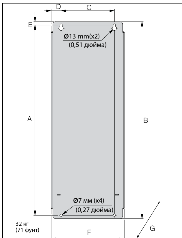
Рис. 14 Устройство Emotron VFX моделей с 48/52-061 по 074 (размер корпуса D), моделей с 69-033 по 69-058, (размер корпуса D69).
