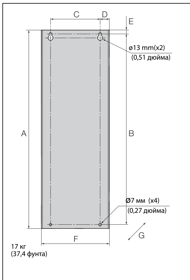
Рис. 12 Устройство Emotron VFX моделей 69-002 — 025 (размер корпуса C69).
