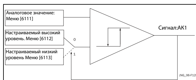
Рис. 132 Аналоговый компаратор гистерезисного типа
