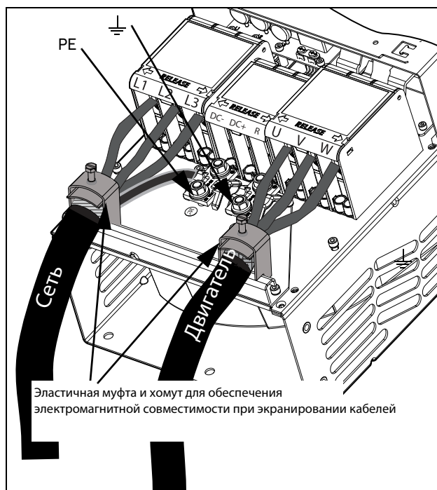
Рис. 38 Подключение сетевого питания и двигателя моделей 48-142 — 48-293 (размеры корпуса E2 и F2) с дополнительными клеммами для опции DC-, DC+ и тормоза (принципиальная схема)
