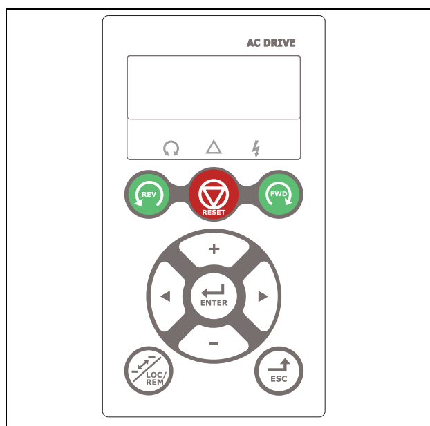
Рис. 151 Панель управления с 4-строчным дисплеем
