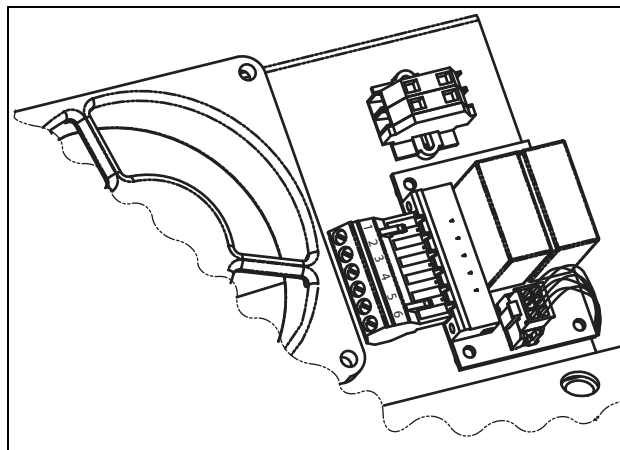
Рис. 160 Подключение дополнительной платы безопасного останова для размера E и больше.
