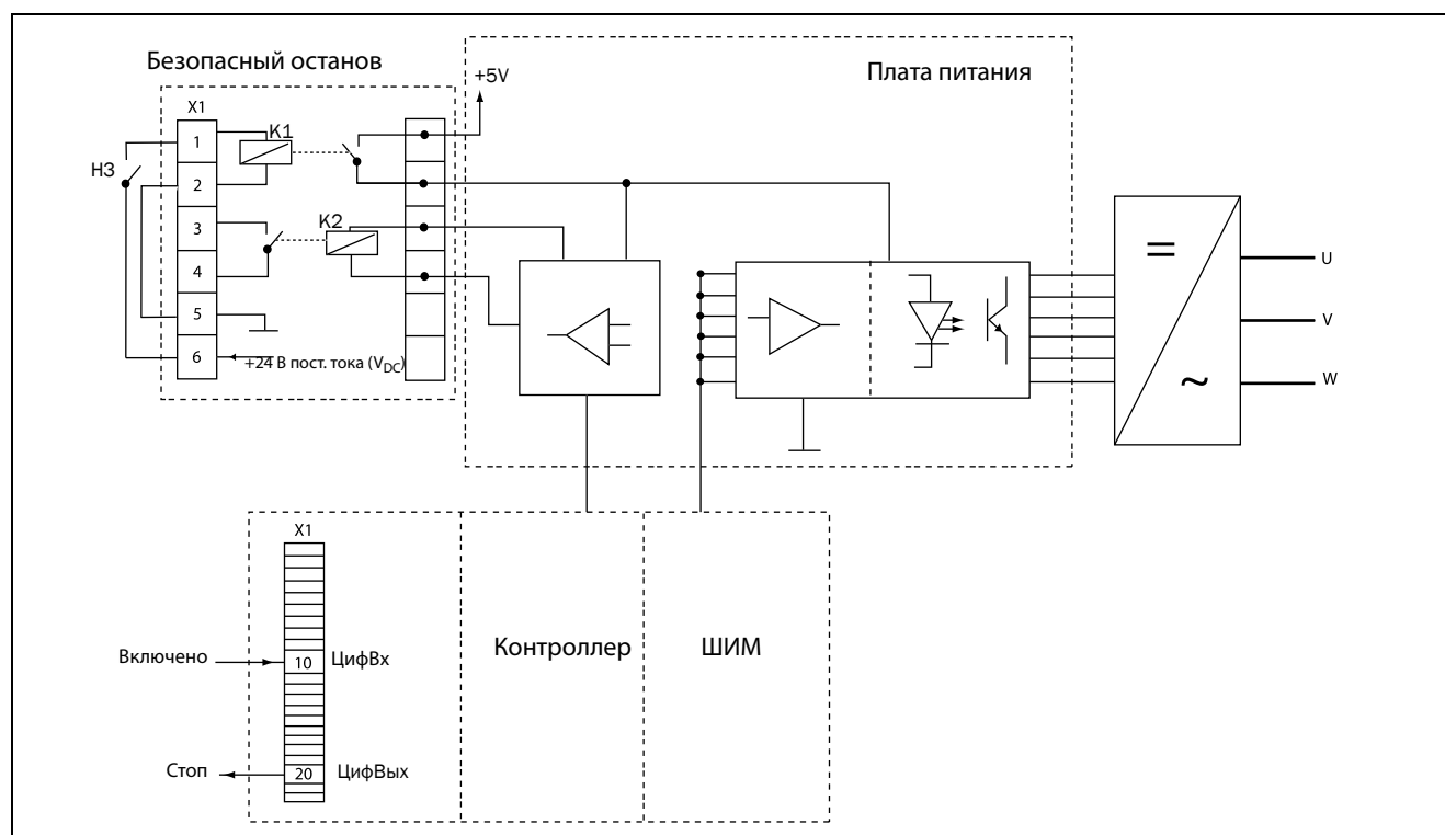
Рис. 161 Подключение функции безопасного останова
