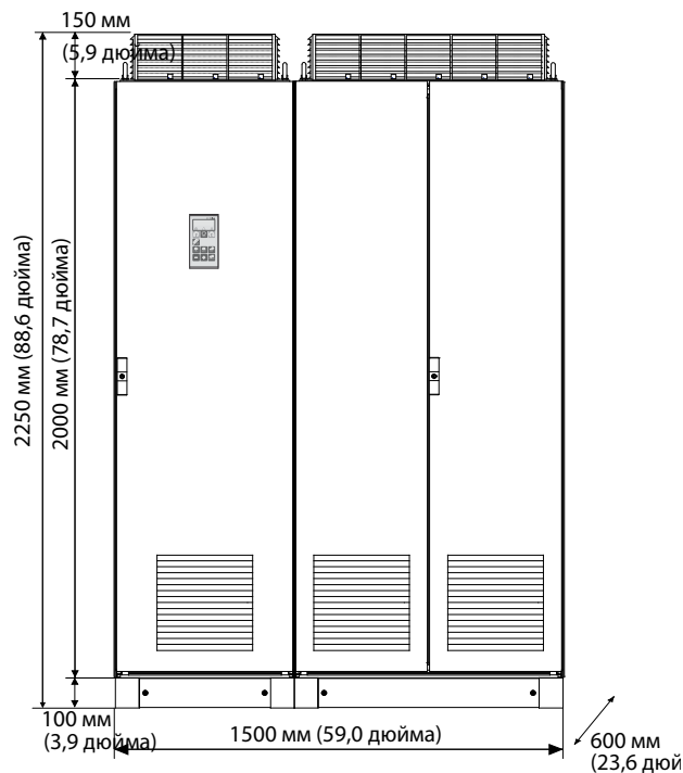
Устройство Emotron VFX48: модели от 1K15 до 1K25 (размер корпуса KA) Устройство Emotron VFX69: модели 905–995 (размер корпуса KA69)
