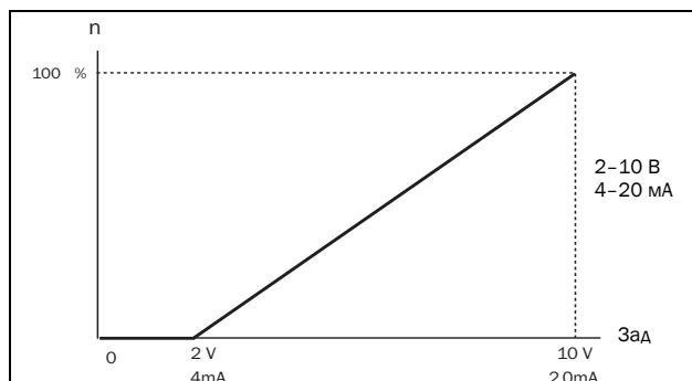
Рис. 128 2–10 В/4–20 мА (реальный ноль)
