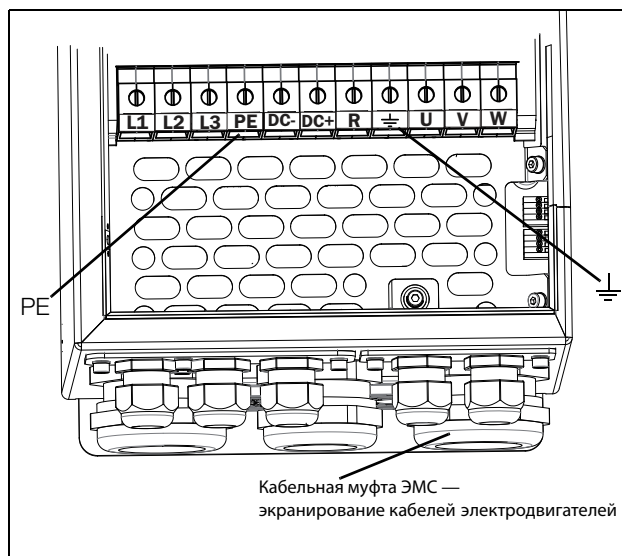
Рис. 35 Подключение сетевого питания и двигателя, модель 061-074, размер корпуса D и моделей 69-033 — 69-058, размер корпуса D69
