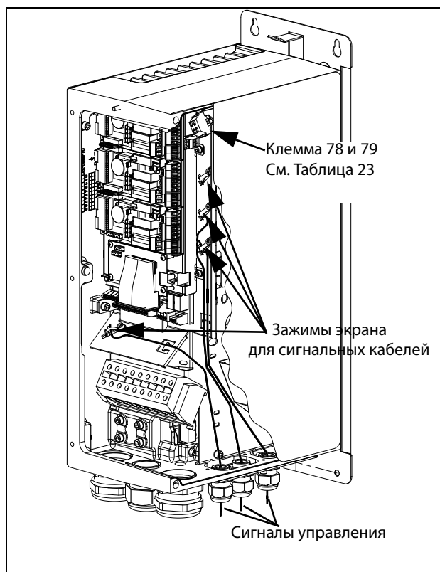
Рис. 59 Подключение кабелей управления, VFX модели от 026 до 046, типоразмер С.
