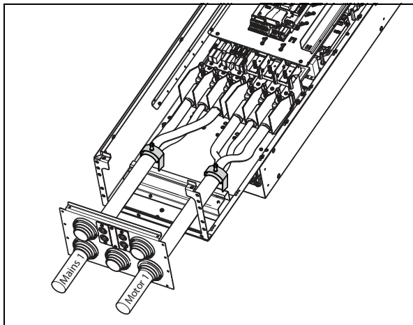
Рис. 46 Снимите верхнюю монтажную рейку.
