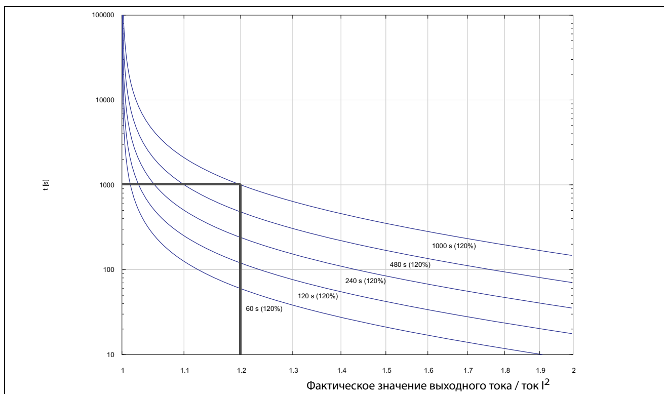
Рис. 95 Функция I^2t
