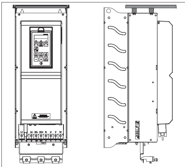
Рис. 162 Дополнительная верхняя крышка, установленная на корпусе размера D2
