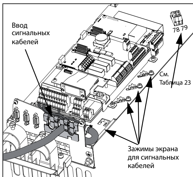
Рис. 60 Подключение кабелей управления, модели, VFX 48-025 — 48-058 с размером корпуса С2 и модели 69-002 — 69-025 с размером корпуса С2 (69)
