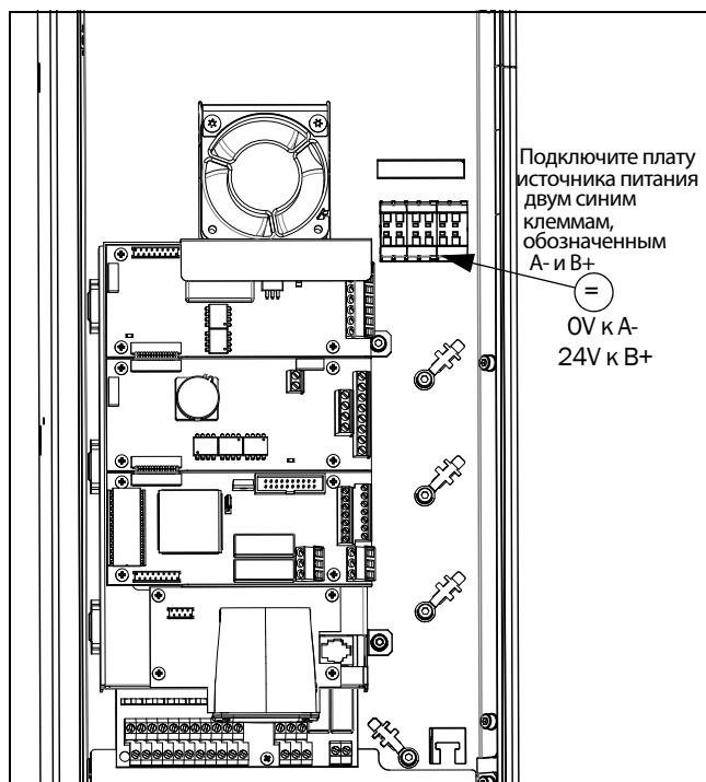
Рис. 158 Подключение опции резервного источника питания для размеров корпуса D, D2, FA, FA2, C69, D69, C2(69) и D2(69).
