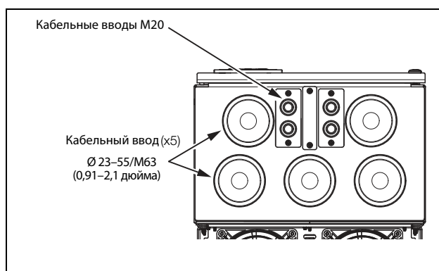
Рис. 26 Кабельный интерфейс для подключения электрической сети, электродвигателя, DC+/DC-, тормозного резистора и связи, устройство Emotron VFX модели 48-365-54 (размер корпуса FA).
