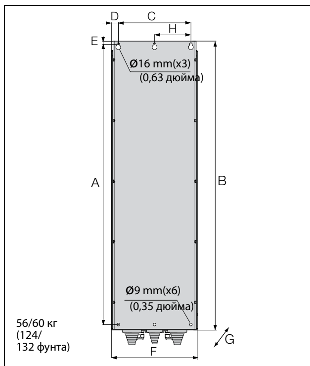
Рис. 18 Устройство Emotron VFX моделей с 48-090 по 175 (размер корпуса E).
