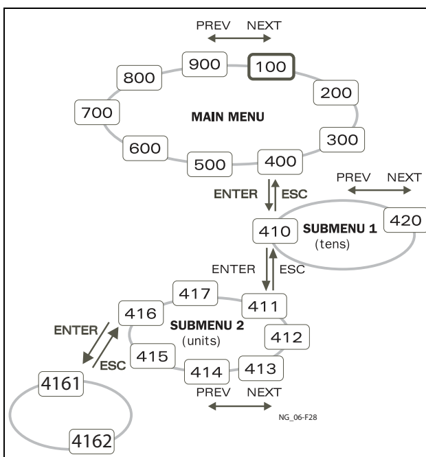
Рис. 90 Структура меню
