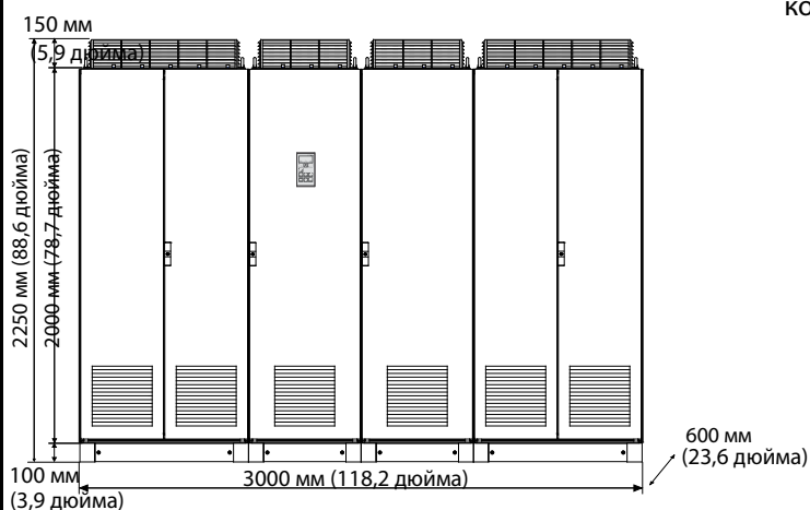
Устройство Emotron VFX48: модель 2K5 (размер корпуса O) Устройство Emotron VFX69: модель 2K0 (размер корпуса O69)
