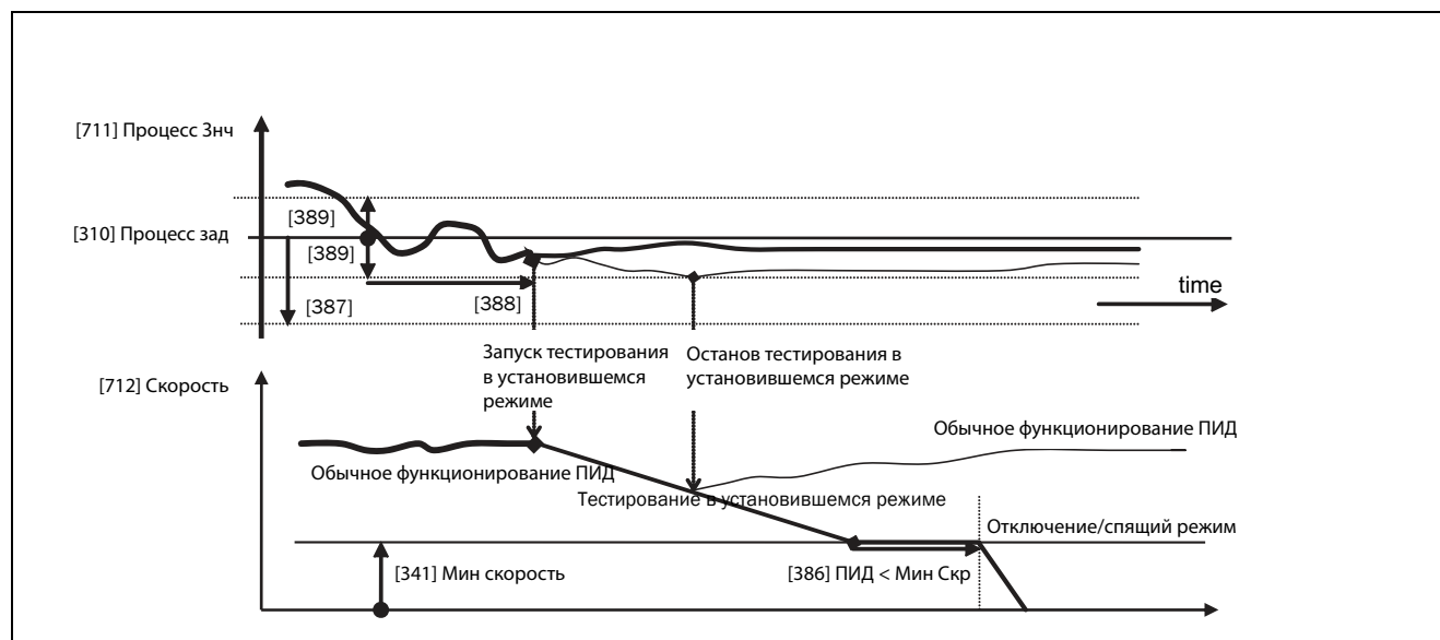
Рис. 114 Тестирование в установившемся режиме
