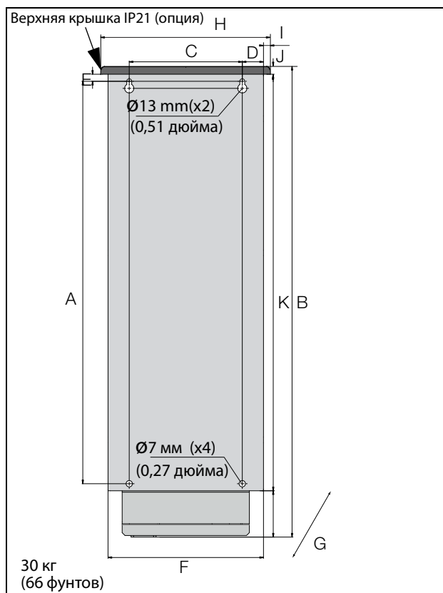
Рис. 16 Устройство Emotron VFX моделей с 48-060 по 48-105 (размер корпуса D2), моделей с 69-033 по 69-058 (размер корпуса D2(69)), вид сзади.
