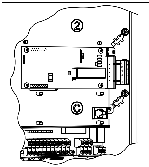
Рис. 159 Подключение опциональной платы безопасного останова для размеров корпуса B-D.
