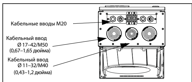
Рис. 19 Кабельный интерфейс для подключения электрической сети, электродвигателя, DC+/DC-, тормозного резистора и связи, устройство Emotron VFX моделей с 48-090 по 175 (размер корпуса E)
