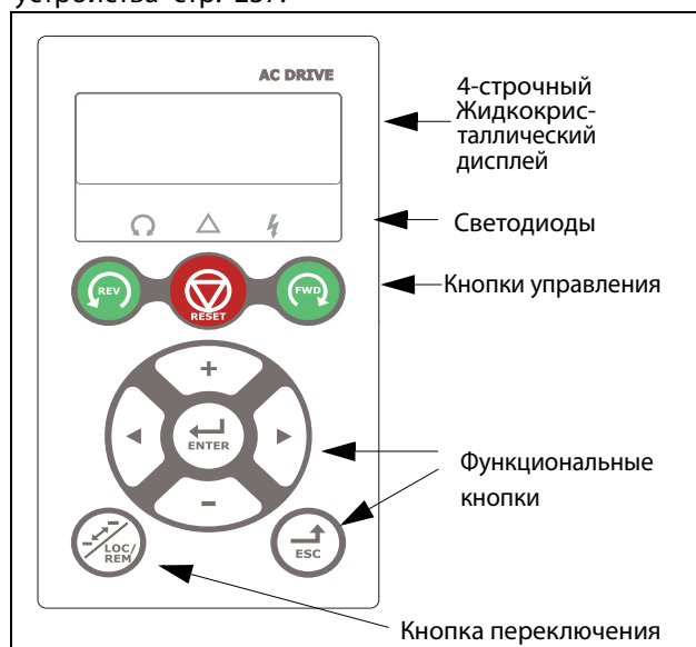
Рис. 78 Панель управления с 4-строчным дисплеем, светодиодные индикаторы и кнопки
