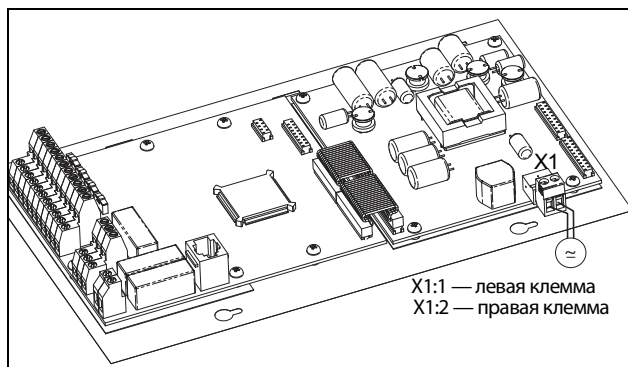
Рис. 157 Подключение опции резервного источника питания для размеров В, С, С2, Е, Е2, F и F2.
