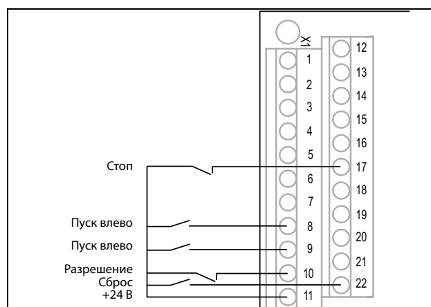
Рис. 72 Пример подключения входов "Пуск/Стоп/Разрешение/Сброс"
