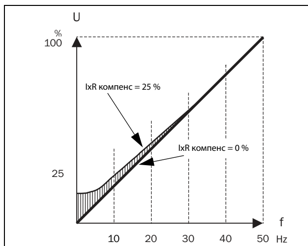
Рис. 108 IxR компенсация при линейной зависимости В/Гц
