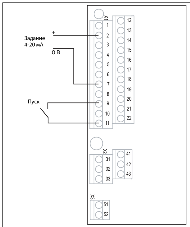
Рис. 68 Подключение
