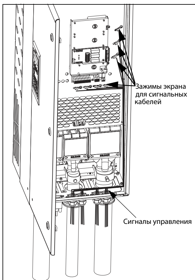
Рис. 63 Подключение кабелей управления, VFX модели от 48-090 до 295 и VFX модели от 69-82 до 200, типоразмер E, F и F69 (принципиальная схема).
