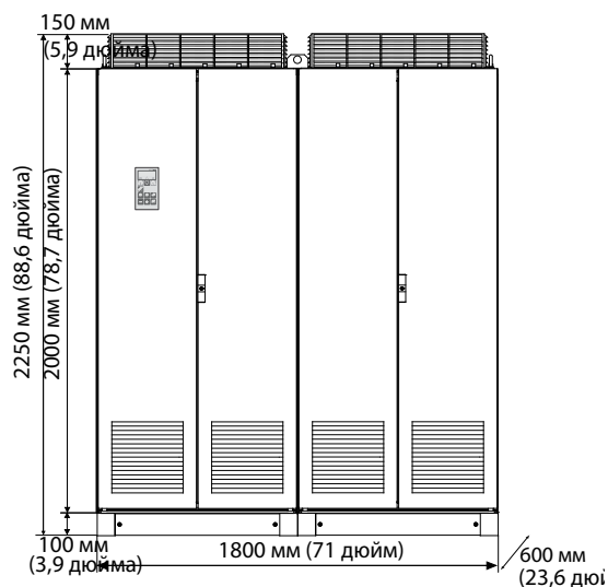
Устройство Emotron VFX48: модели от 1K35 до 1K5 (размер корпуса KA) VFX69: модель 1K2 (размер корпуса K69)
