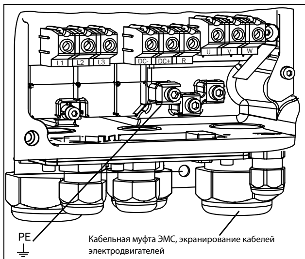
Рис. 31 Подключение сетевого питания и двигателя модели 003-018, размер корпуса B.
