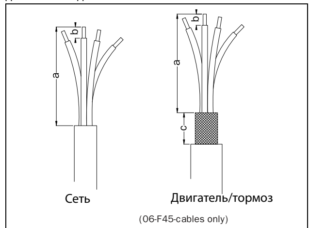
Рис. 53 Длина зачистки кабелей
