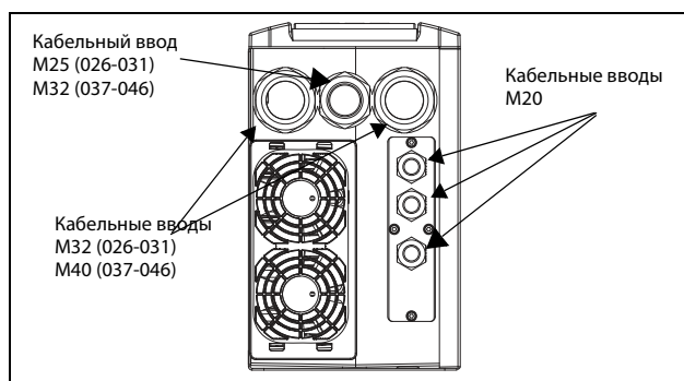
Рис. 9 Кабельный интерфейс для подключения электрической сети, электродвигателя и управления, устройство Emotron VFX моделей 48/52-026 — 046 (размер корпуса C).
