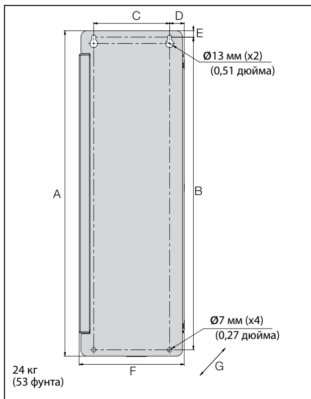
Рис. 8 Устройство Emotron VFX моделей 48/52-026 — 046 (размер корпуса C).
