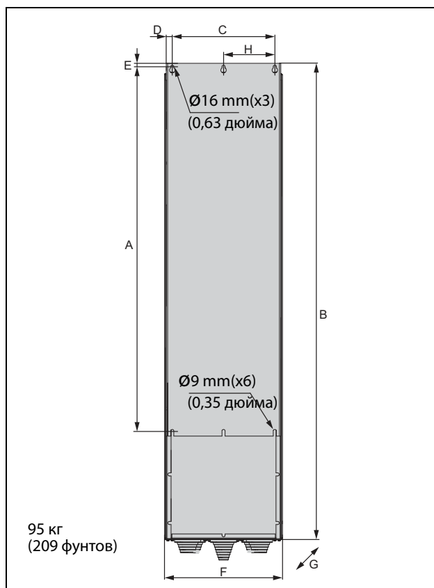
Рис. 25 Устройство Emotron VFX модели 48-365-54 (размер корпуса FA).
