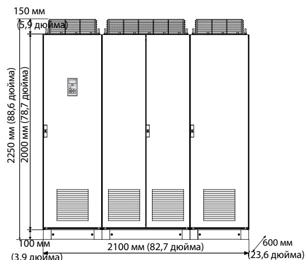
Устройство Emotron VFX48: модель 1K75 (размер корпуса L) Устройство Emotron VFX69: модель 1K4 (размер корпуса L69)
