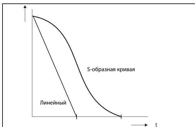
Рис. 102 Форма кривой торможения
