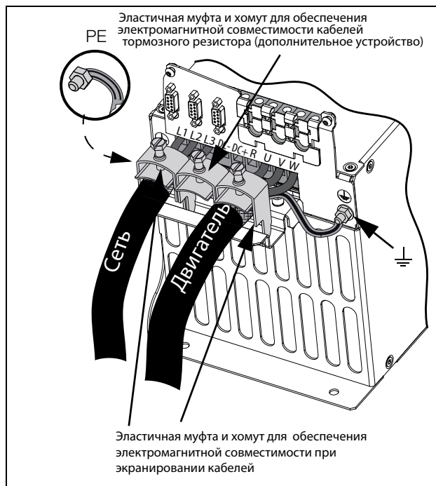
Рис. 34 Подключение сетевого питания и двигателя моделей 48-025 — 48-058, размер корпуса C2 и моделей 69-002 — 69-025, размер корпуса C2(69)
