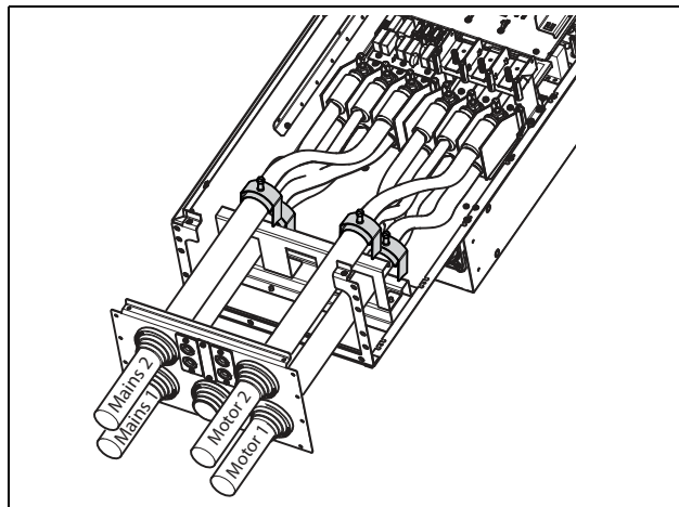
Рис. 48 Все кабели и кабельные зажимы подключены.
