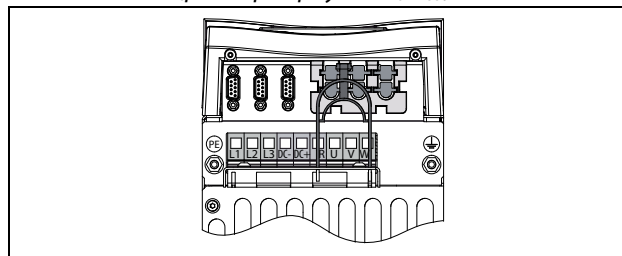
Рис. 10 Устройство Emotron VFX моделей 48-025 по 48-058 (размер корпуса C2), моделей 69-002 — 69-025 (размер корпуса C2(69)), вид сзади.
