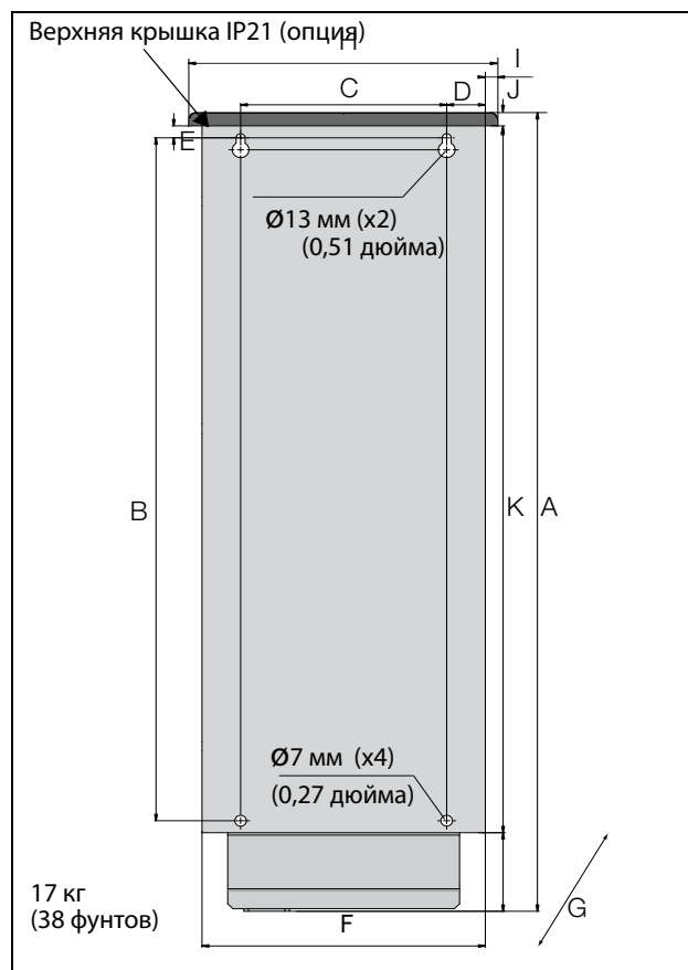
Рис. 10 Устройство Emotron VFX моделей 48-025 по 48-058 (размер корпуса C2), моделей 69-002 — 69-025 (размер корпуса C2(69)), вид сзади.
