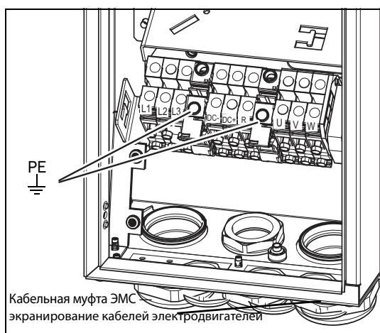
Рис. 33 Подключение сетевого питания и двигателя модели 002-025, размер корпуса C69
