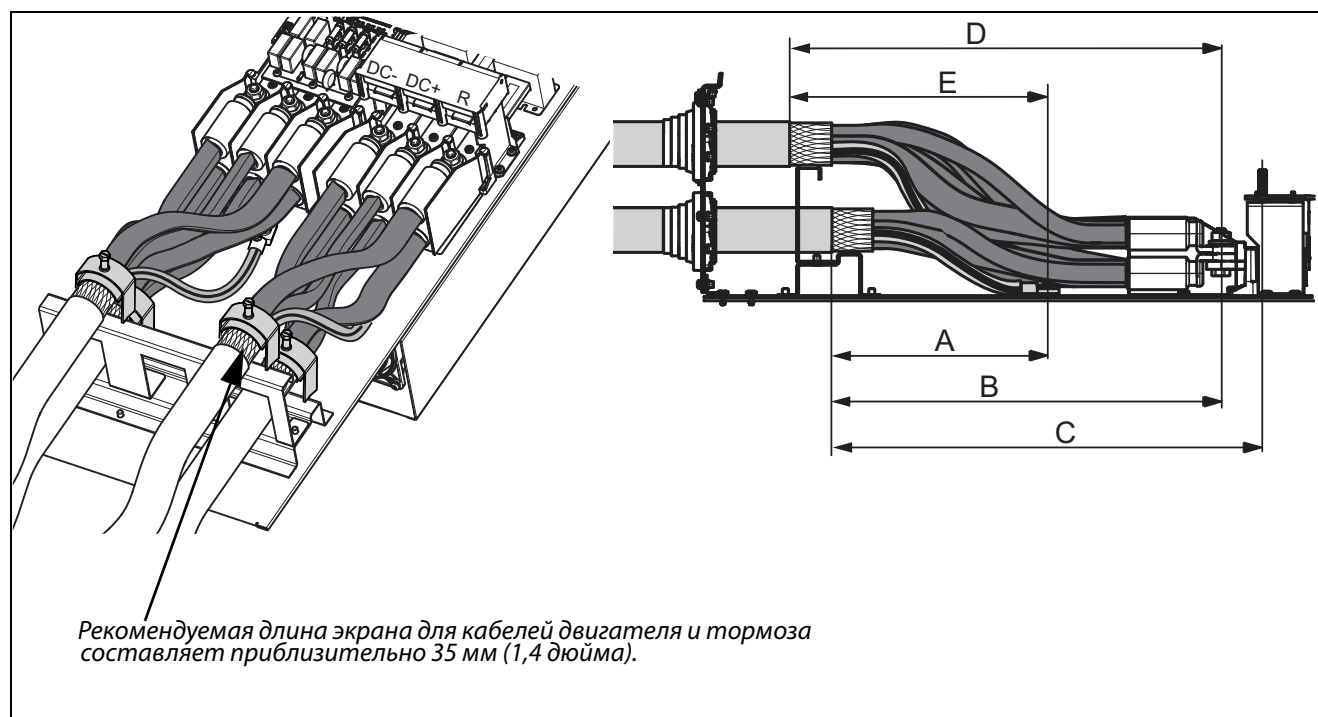
Рис. 55 Расстояния от кабельного зажима до соединительных болтов размера FA
